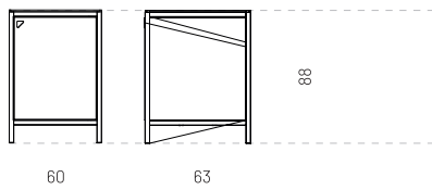
Workbench | Ty door Werkbank | Ty-Tür
